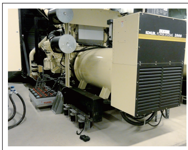
發電機安裝YS-EA橡膠式擊震器
