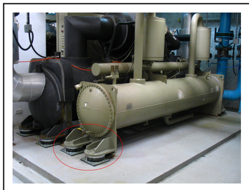
冰機安裝YS-K氣墊式避振器
