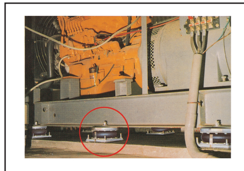
發 電 機
