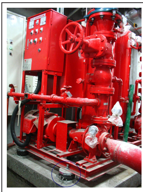
消防泵安裝YS-K氣墊式避振器
