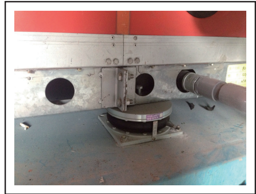
空調箱安裝YS-K氣墊式避振器
