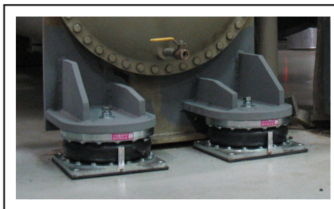
冰水主機安裝YS-K氣墊式避振器
