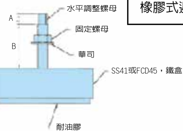
沖床安裝YS-SS橡膠式避振器
